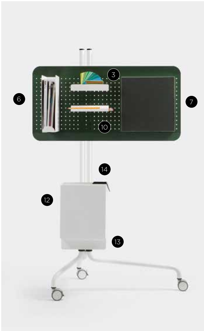
1 ISLAND-01 Isla de trabajo portátil Free standing portable device Île de travail mobile Mobile Arbeitsinsel 633 x 420 x 1502 mm. 24-15/16" x 16-9/16" x 59-1/8"
